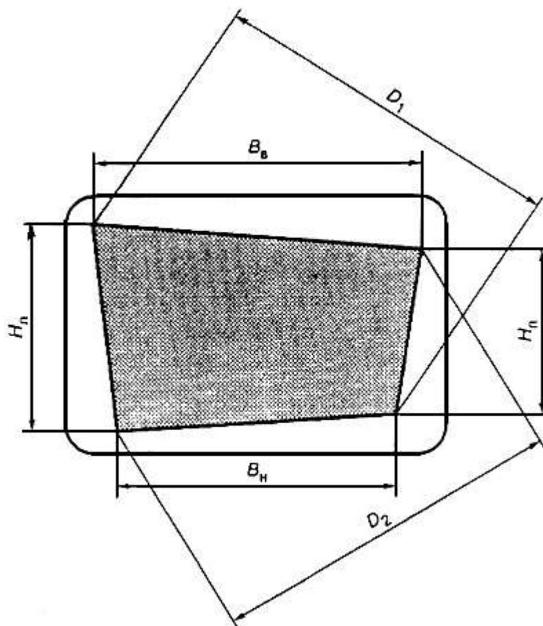
Рисунок 6 - Определение отклонения рабочего поля от прямоугольной формы
