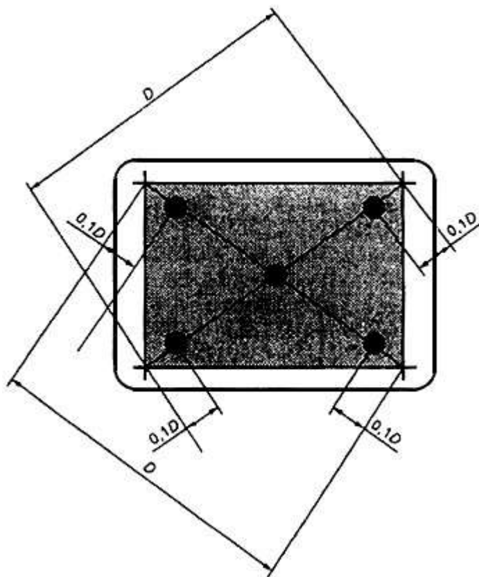
Рисунок 1 - Участки экрана, предусмотренные для измерения параметров изображения
