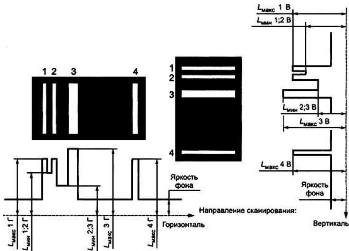
Рисунок 2 - Расположение штрихов и профили яркости тест-изображения
