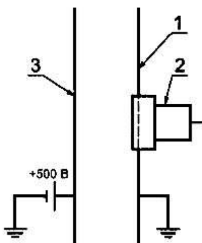
1 - измерительная пластина; 2 - измеритель напряженности поля; 3 - контрольная пластина
