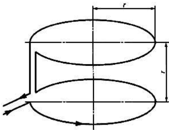
Рисунок Б.1 - Схема катушки Гельмгольца
