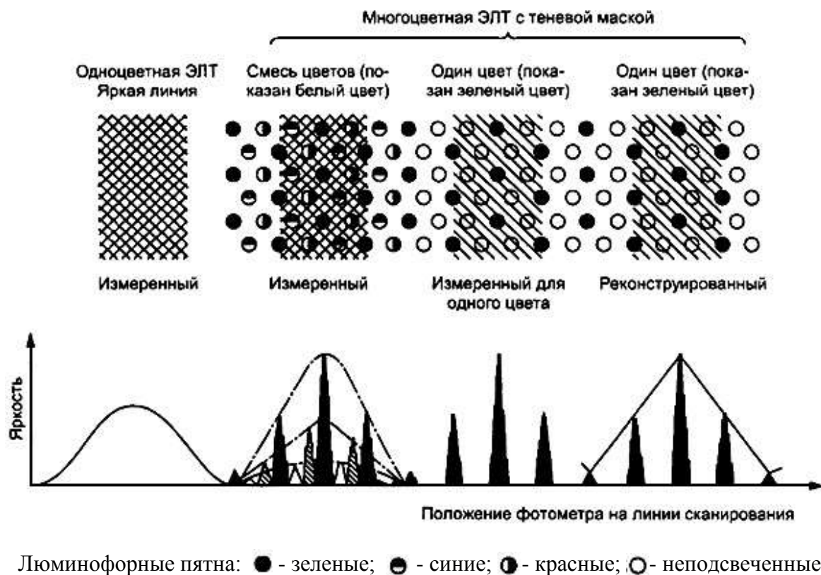
Рисунок Г.1 - Построение профиля яркости детали изображения
